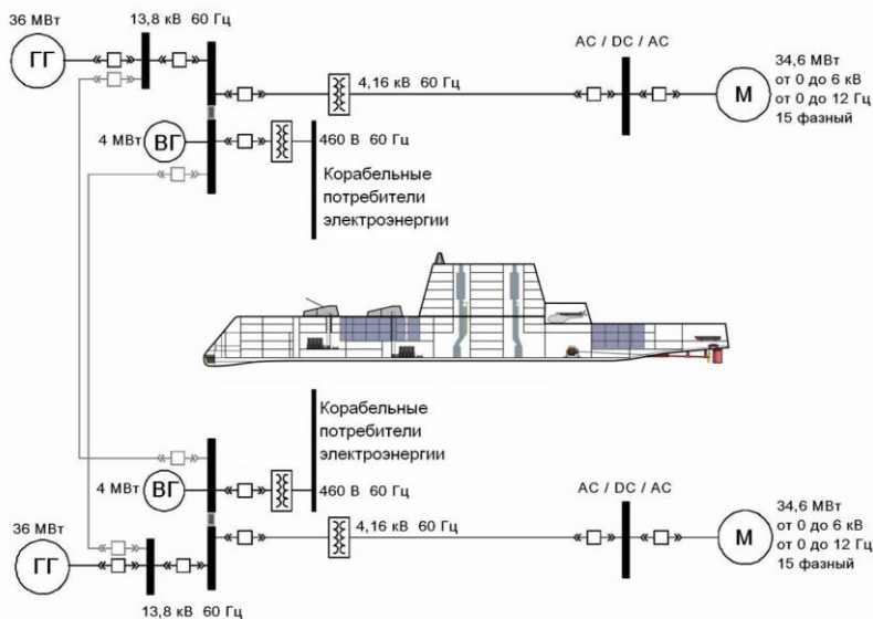
Рис. 1. Схема ЭЭС эсминца типа Zumwalt
