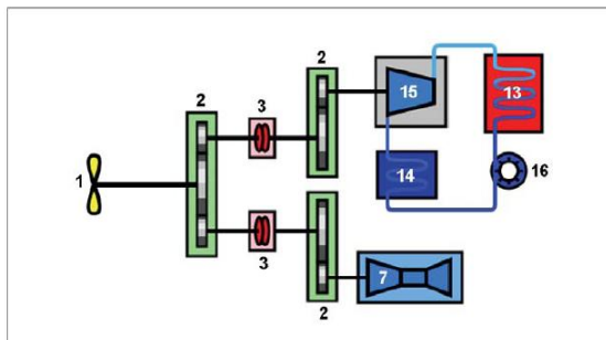
ЭУ по схеме COSAG
