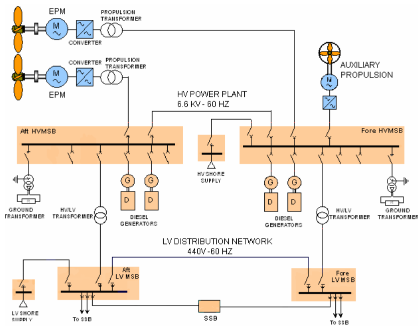
Рис. 2. Схема ЭЭС фрегата типа FREMM
